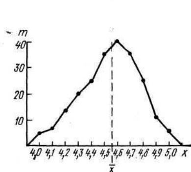
Рис. 1. Полигон распределения признака: ширина горла сосудов (по частотам)
