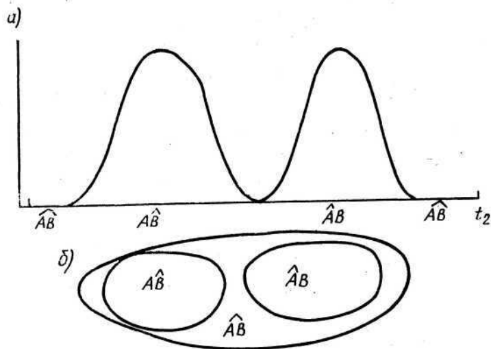
Рис. 19. Интерпретация случая 9 зависимости между качественными признаками:
