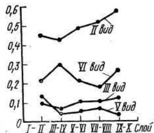
Рис. 4. Полигон распределения долей керамики различного вида в поселке Змейском
