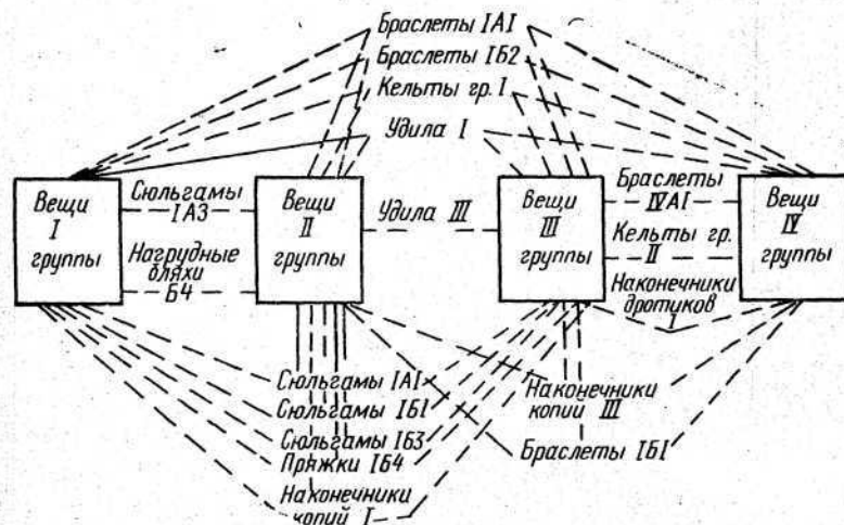
Рис. 24. Граф сильных связей между видами вещей из Безводнинского могильника (по Ю. А. Краснову)
