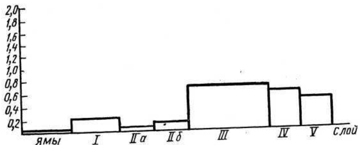
Рис. 6. Гистограмма распределения амфор в Саркеле-Белой Веже
