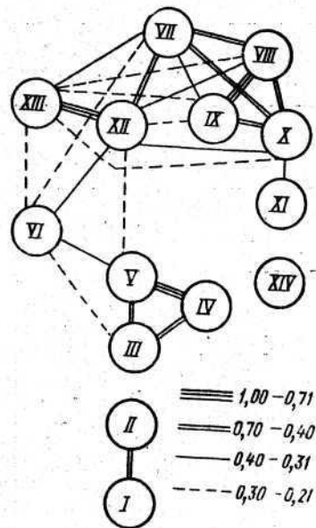
Рис. 21. Граф сходства объектов-крышек из Пенджикента
