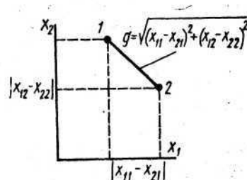
Рис. 20. Вычисление евклидова расстояния между двумя объектами
