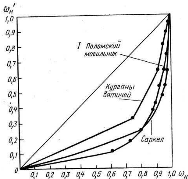
Рис. 3. Кривые Лоренца для распределения бус по погребениям
