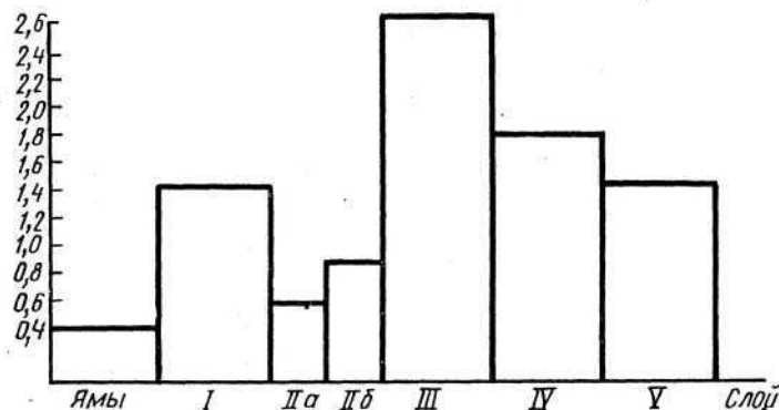
Рис. 5. Гистограмма распределения амфор в Саркеле-Белой Веже
