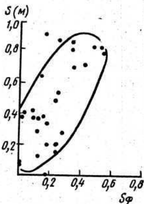
Рис. 26. Корреляция между S(\phi) и S(m) для культур бронзового века (по Е. Н. Черныху)
