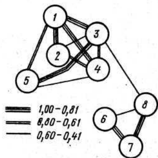
Рис. 25. Граф сходства между культурами по химико-технологическим признакам (по Е. Н. Черныху)
