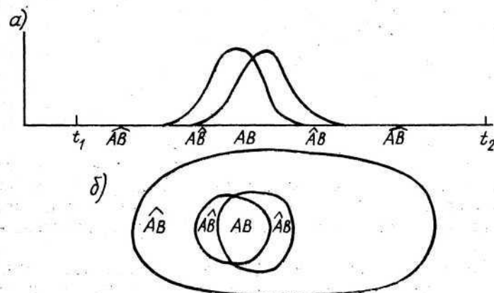
Рис. 16. Интерпретация случая 6 зависимости между качественными признаками:
