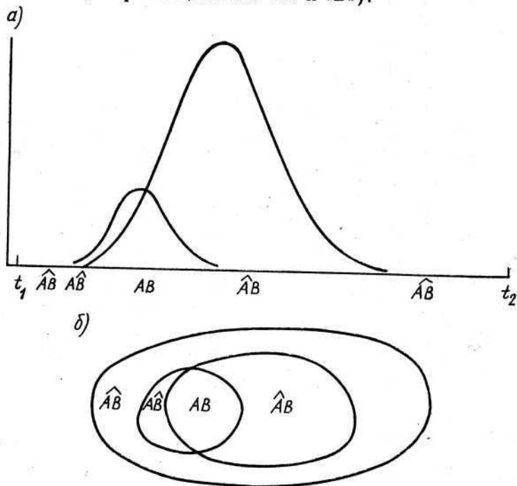
Рис. 13. Интерпретация случая 3 зависимости между качественными признаками:
