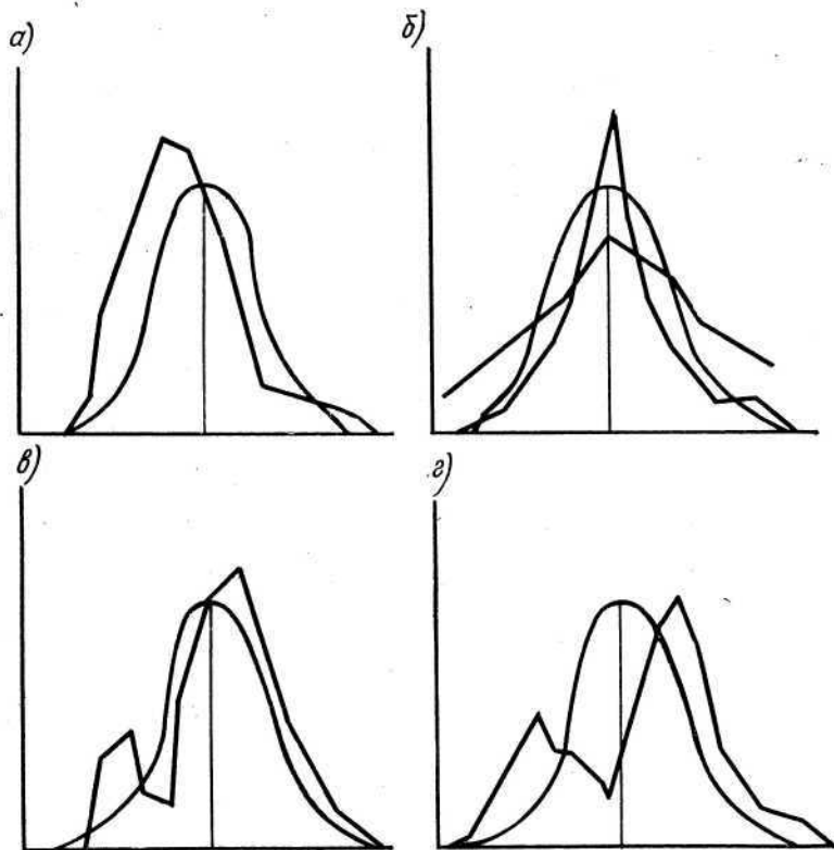
Рис. 9. Отклонения эмпирического распределения от нормального:
