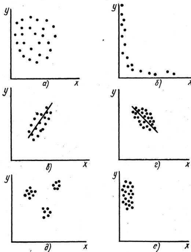
Рис. 10. Различные виды зависимости между количественными признаками:
