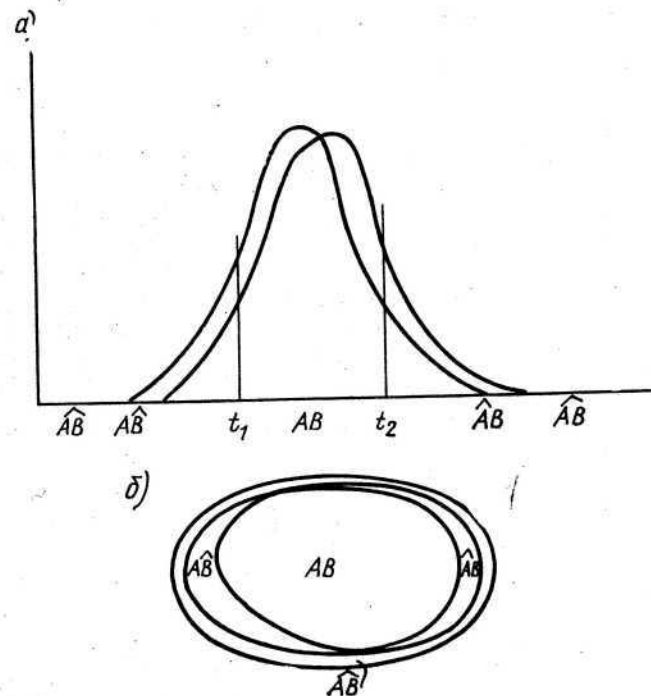
Рис. 14. Интерпретация случая 4 зависимости между качественными признаками:
