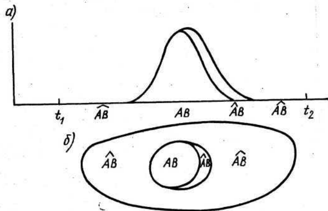
Рис. 17. Интерпретация случая 7 зависимости между качественными признаками:
