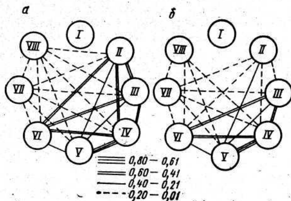
Рис. 27. Граф связей между признаками для бус Северного Кавказа:
