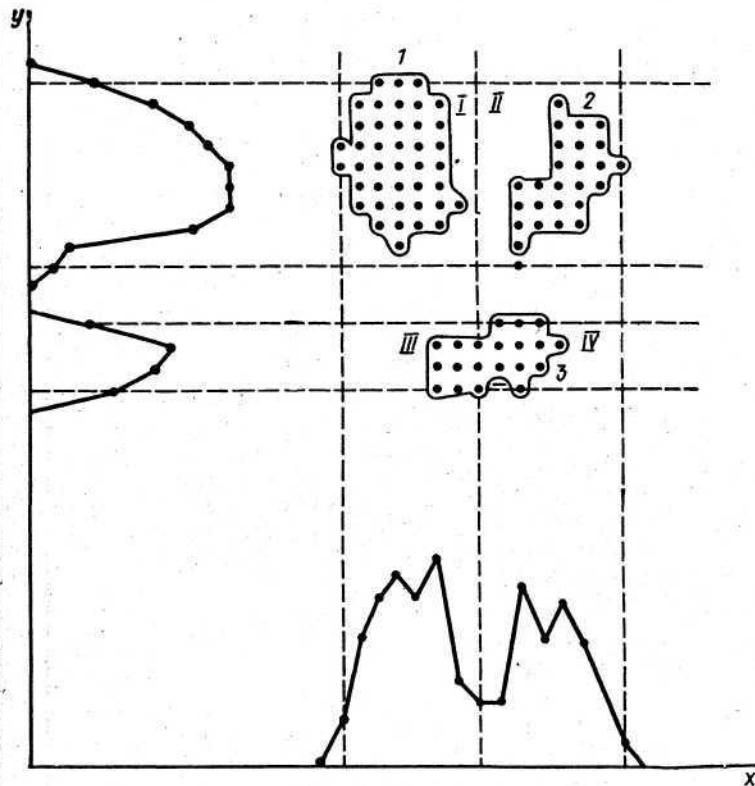
Рис. 31. Соотношение групп, определенных по интервалам признаков и действительной группировкой объектов
