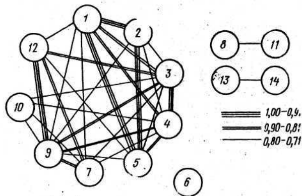
Рис. 29. Граф связей признаков у кувшинов из нижеволожских городищ XIV в.
