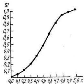
Рис. 2. Кумулята того же распределения
