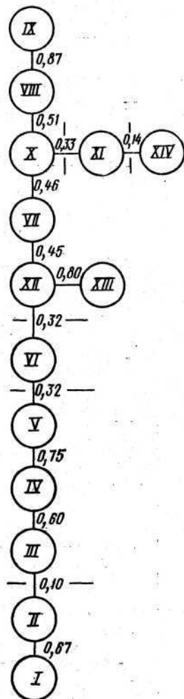
Рис. 22. Граф сходства объектов-крышек из Пенджикента (по методу корреляционных плеяд)
