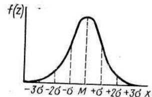
Рис. 8. Кривая нормального распределения
