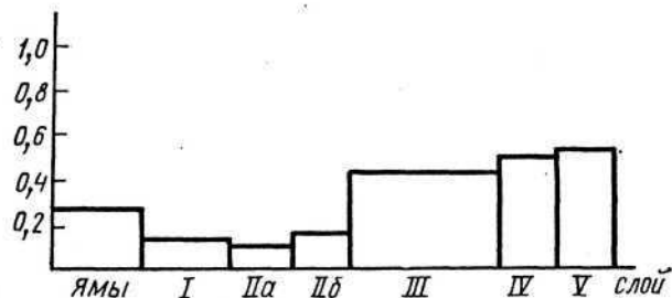
Рис. 7. Гистограмма распределения амфор в Саркеле-Белой Веже
