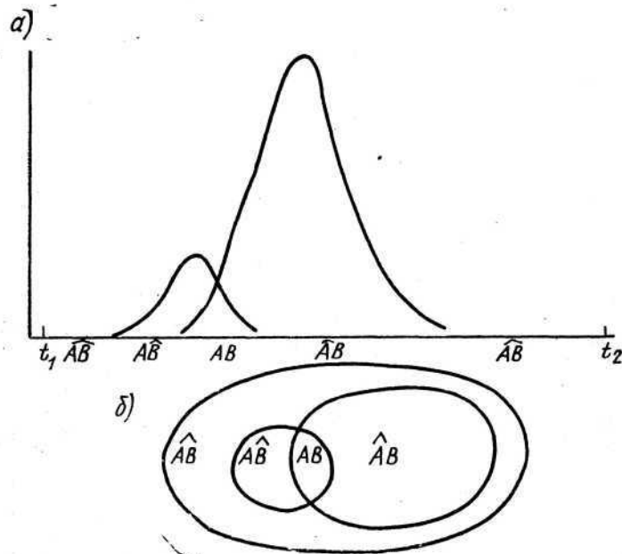
Рис. 12. Интерпретация случая 2 зависимости между качественными признаками:
