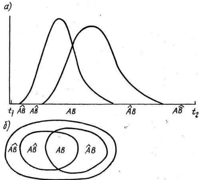
Рис. 11. Интерпретация случая 1 зависимости между качественными признаками:
