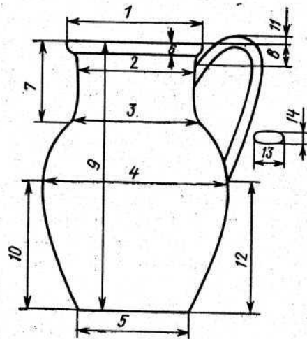
Рис. 28. Количественные (мерные) признаки у кувшинов из нижеволжских городищ XIV в.
