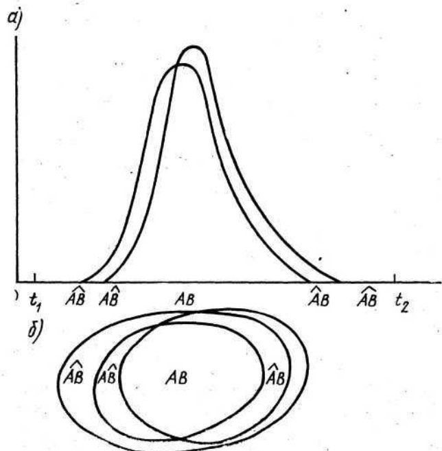
Рис. 15. Интерпретация случая 5 зависимости между качественными признаками:
