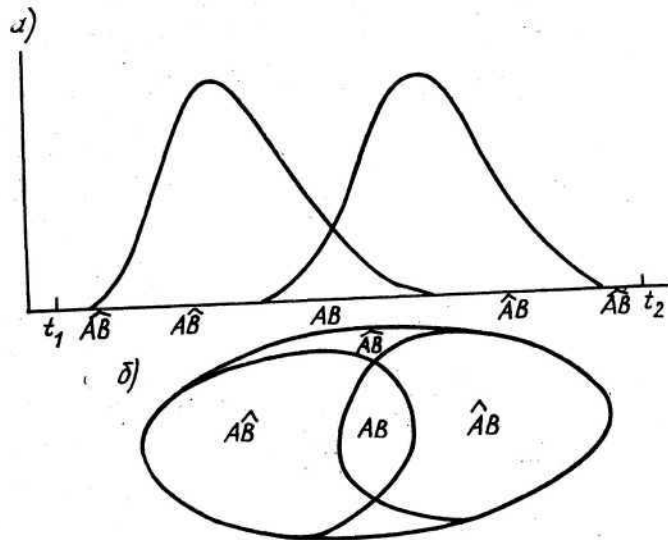
Рис. 18. Интерпретация случая 8 зависимости между качественными признаками:
