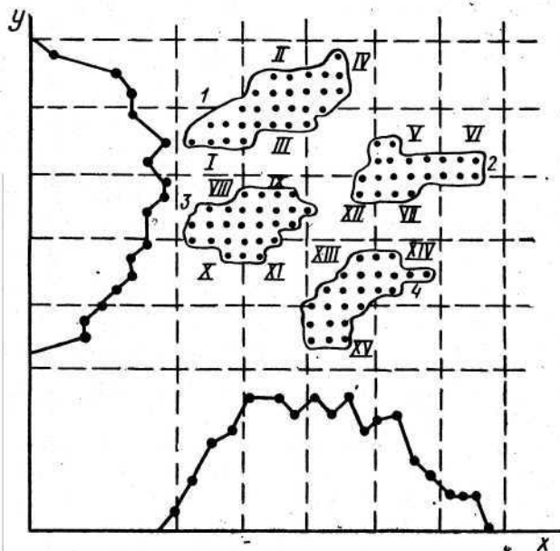
Рис. 30. Соотношение групп, определенных по интервалам признаков и действительной группировкой объектов
